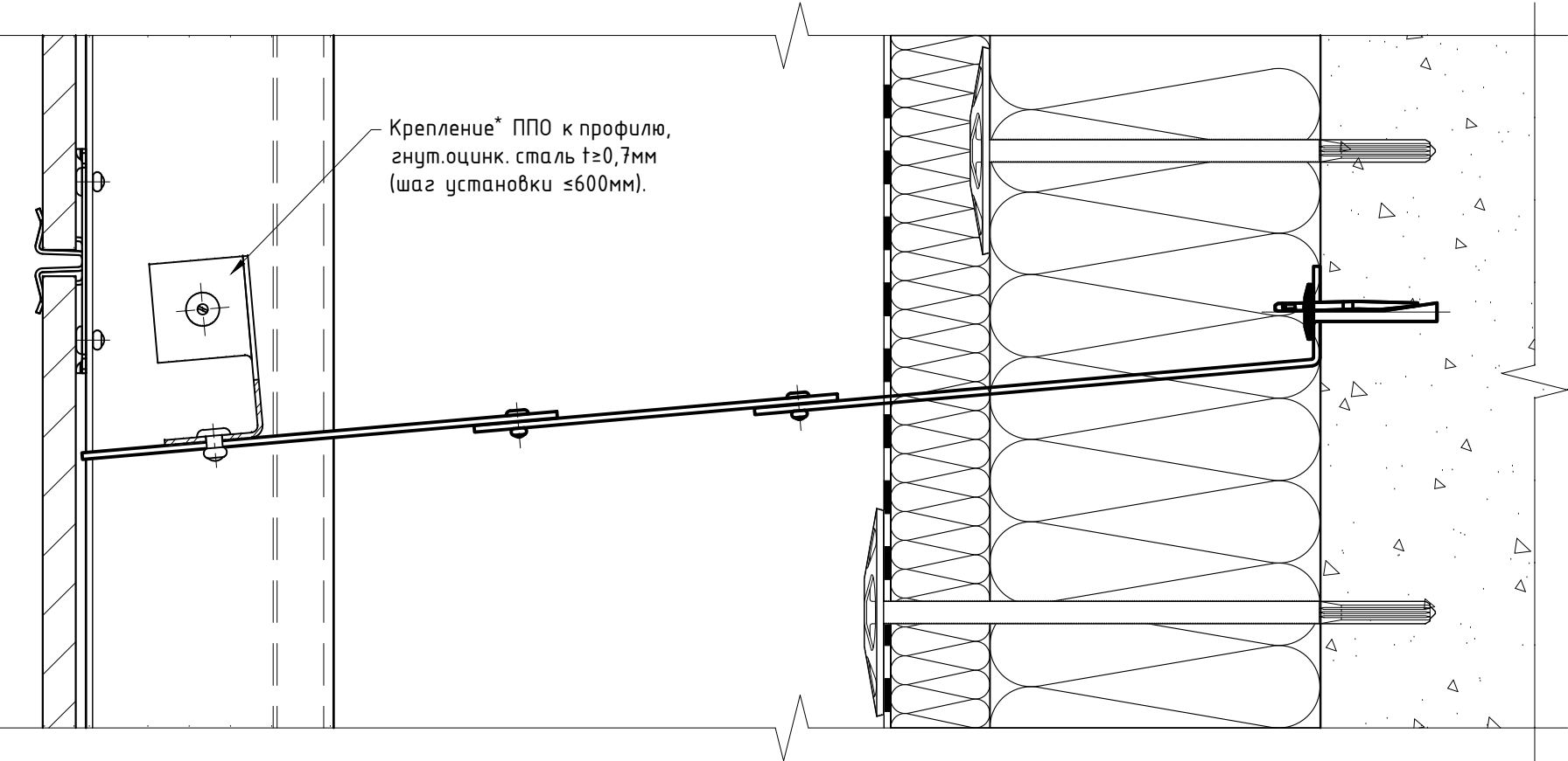
Горизонтальная ППО, а так же сечение по основному узлу для вертикальных элементов фасада (см. предыдущий лист).
