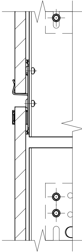
Фрагмент №1 (крепление на рядовой комбинированный кляммер MFT-CVMS A2, вид кляммера показан концептуально)
