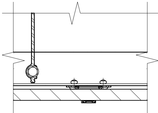
Фрагмент №1 (промежуточное крепление плиты по горизонтальному шву облицовки)
