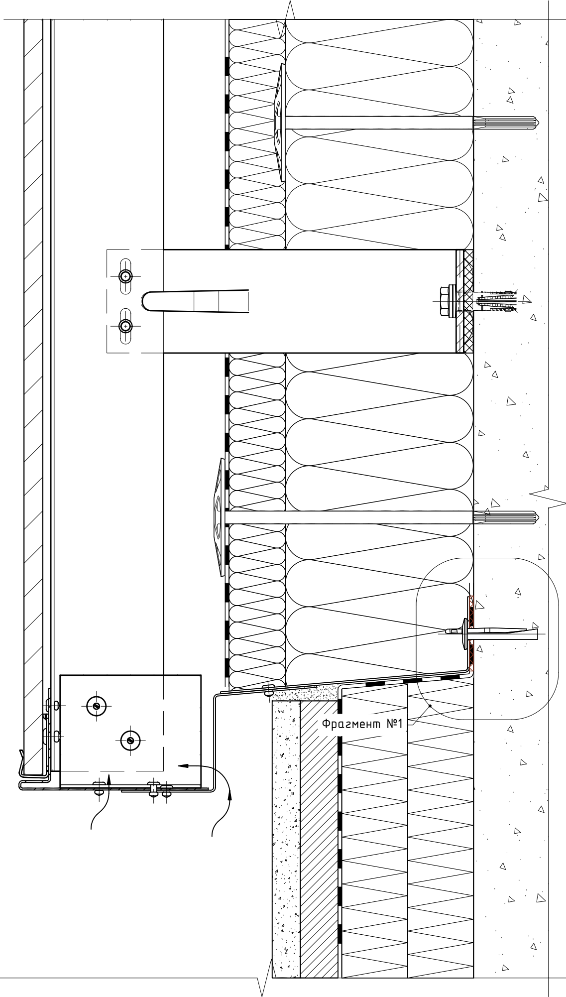
Фрагмент №1 (дополнительный вариант примыкания цоколя к НВФ в зоне строительного основания)
