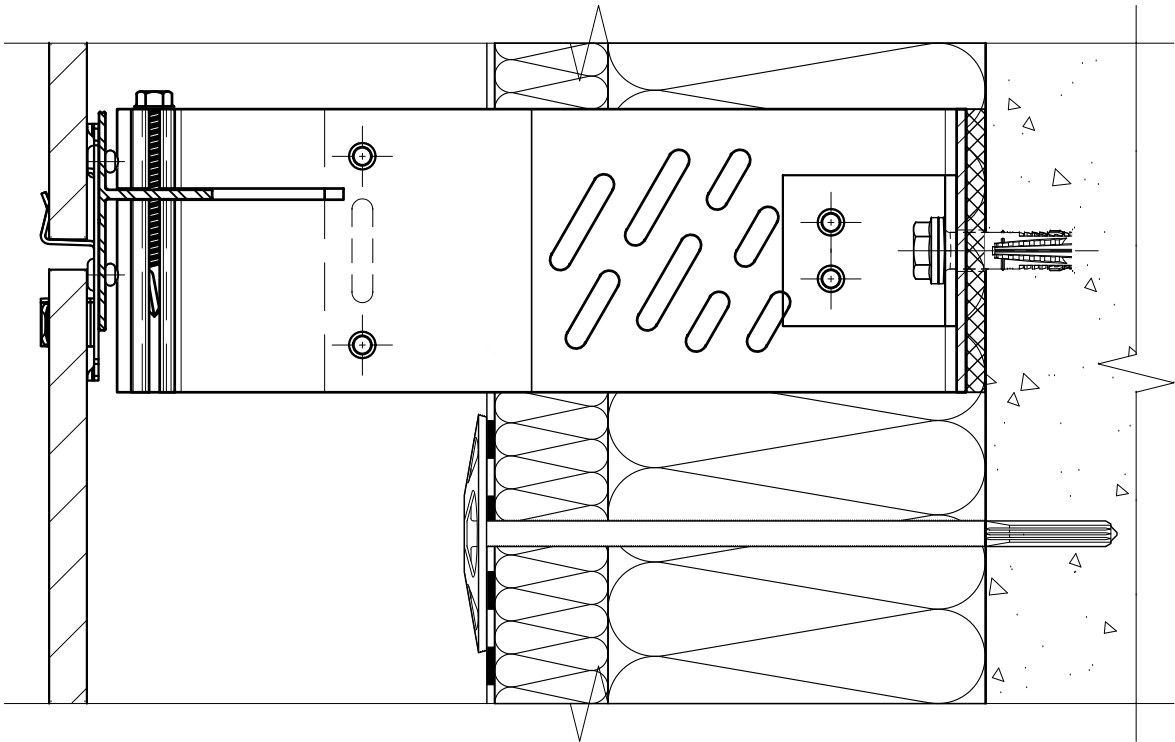
Фрагмент №1 (энергоэффективная система, крепление на рядовой комбинированный кляммер MFT-CVMS A2, вид кляммера показан концептуально)
