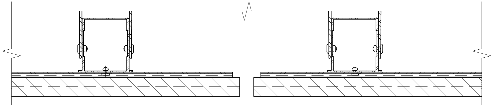
Фрагмент №1 (элементы "Heavy", скрытое крепление на кляммер-шины)
