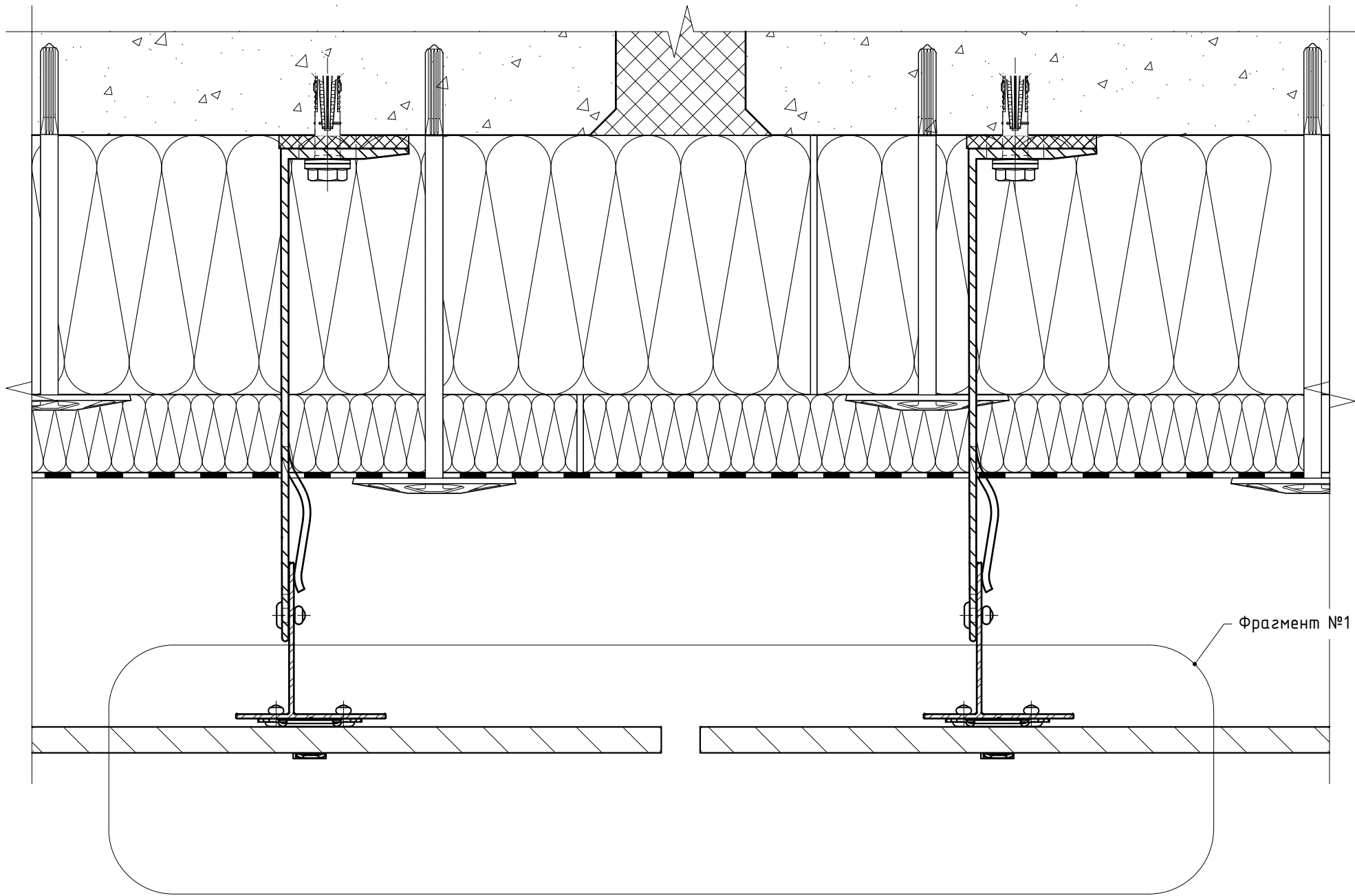
Фрагмент №1 (элементы "Heavy", скрытое крепление на кляммера (в пропилы))
