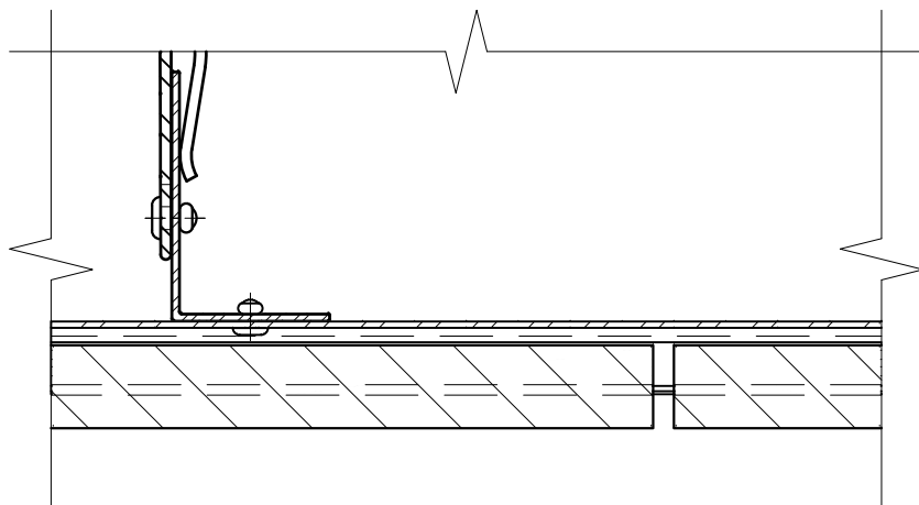
Фрагмент №1 (промежуточное крепление кляммер-шин)
