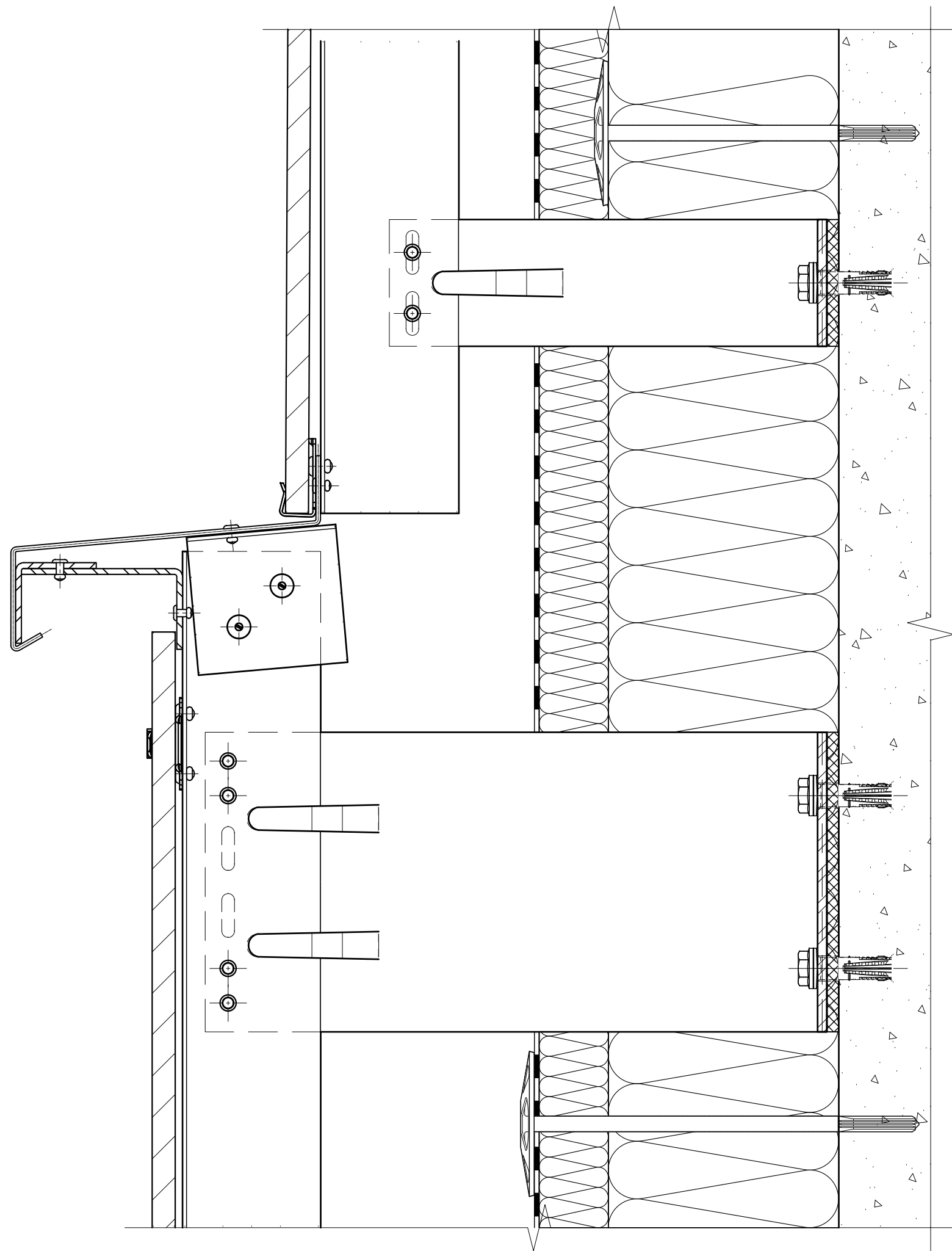
7.12. Организация перепада плоскостей облицовки: вертикальный разрез, видимое крепление на кляммера, вариант №1.
