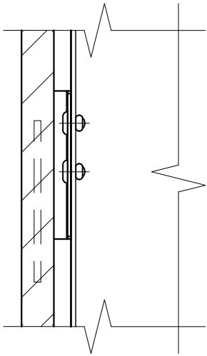
Фрагмент №1 (промежуточное крепление плиты по вертикальному шву облицовки вне зоны стыковки вертикальных направляющих)
