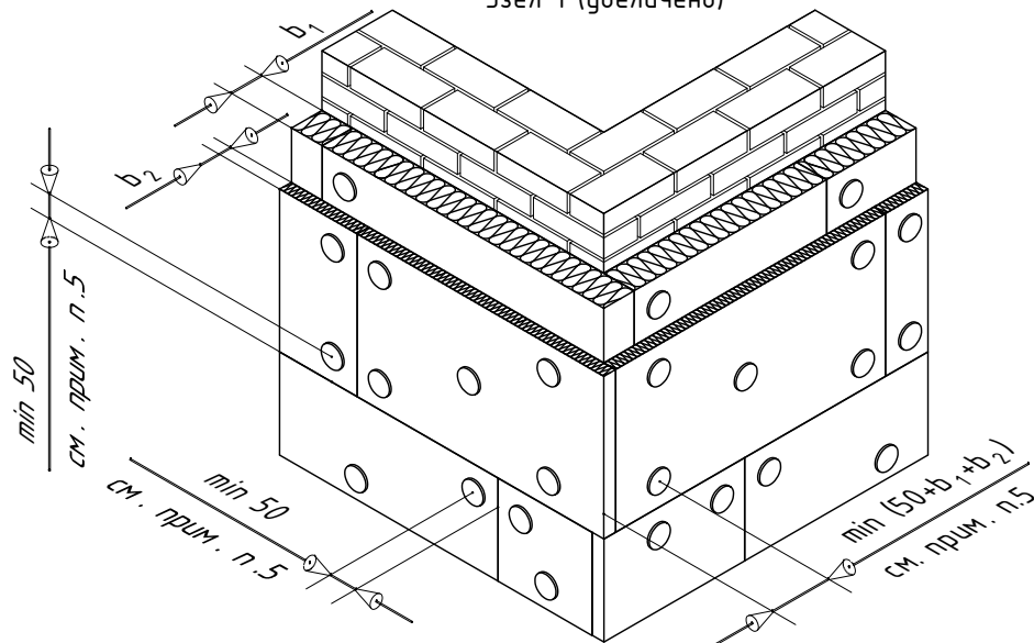
Узел 1 (увеличено)
