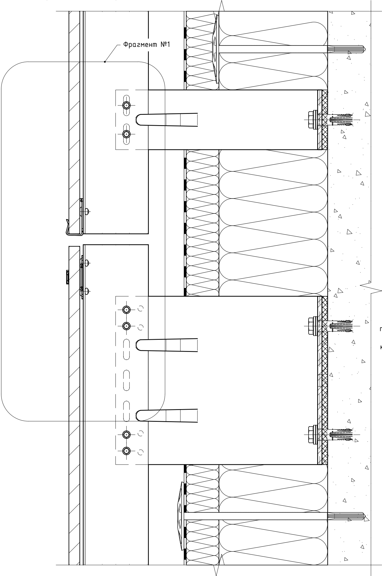
7.2. Вертикальный разрез: элементы "Light", стандартная схема расположения элементов системы ("рядовая"), видимое крепление на клеммера.
