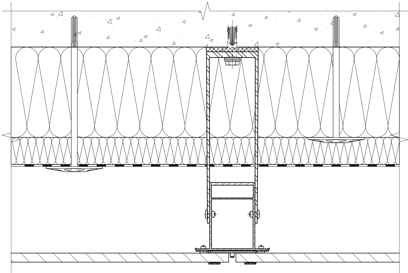
Горизонтальный разрез: элементы "Heavy", видимое крепление на кляммера.
