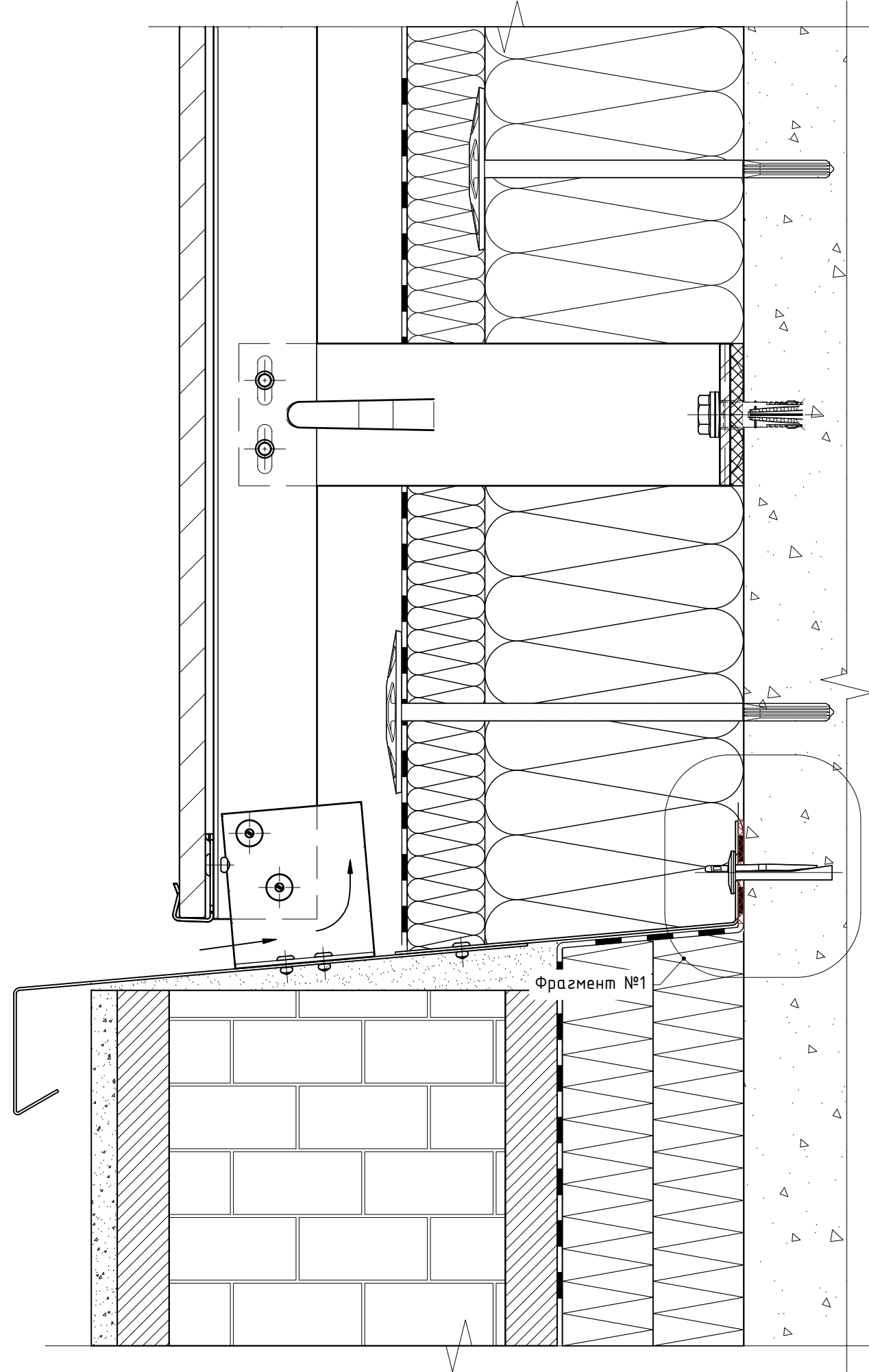
Фрагмент №1 (дополнительный вариант примыкания цоколя к НВФ в зоне строительного основания)
