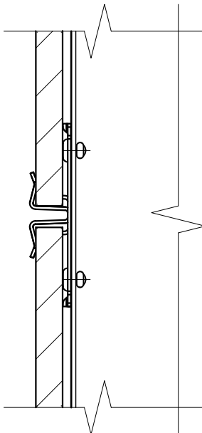
Фрагмент №1 (промежуточное крепление плиты по горизонтальному шву облицовки вне зоны стыковки вертикальных направляющих)
