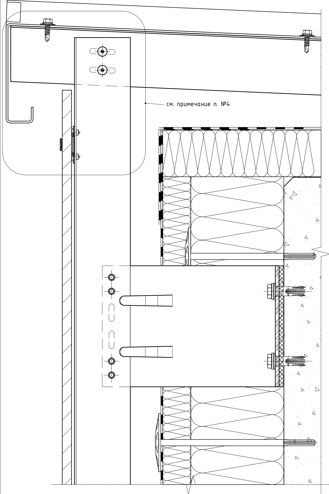
7.9. Примыкание к парапету: вариант крепления парапетной крышки, элементы "Light", вертикальная схема расположения элементов системы, видимое крепление на кляммера.
