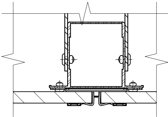
Фрагмент №1 (крепление на рядовой комбинированный кляммер MFT-CVMS A2, вид кляммера показан концептуально)
