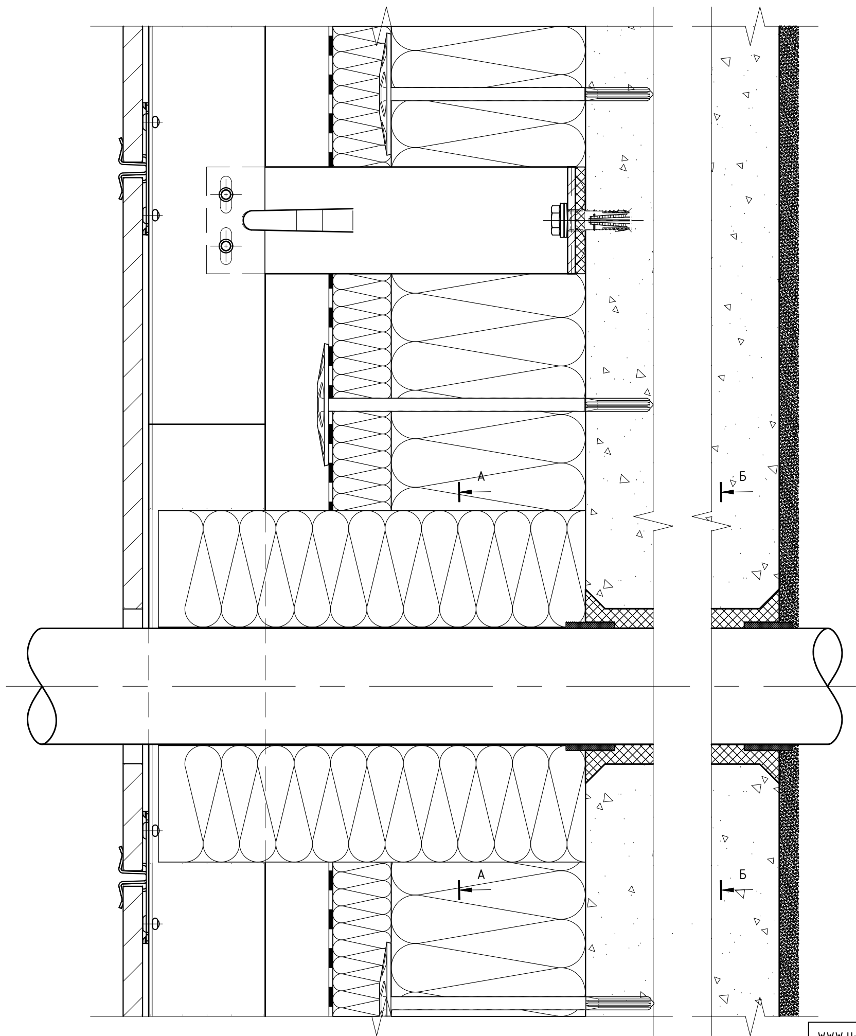
7.11. Ввод коммуникаций: элементы "Light", вертикальная схема расположения элементов системы, видимое крепление на кляммера.
