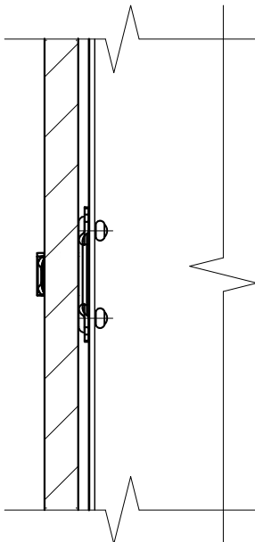
Фрагмент №1 (промежуточное крепление плиты по вертикальному шву облицовки, дополнение к стандартным решениям для площадок с расчетной сейсмичностью 7 и более баллов)
