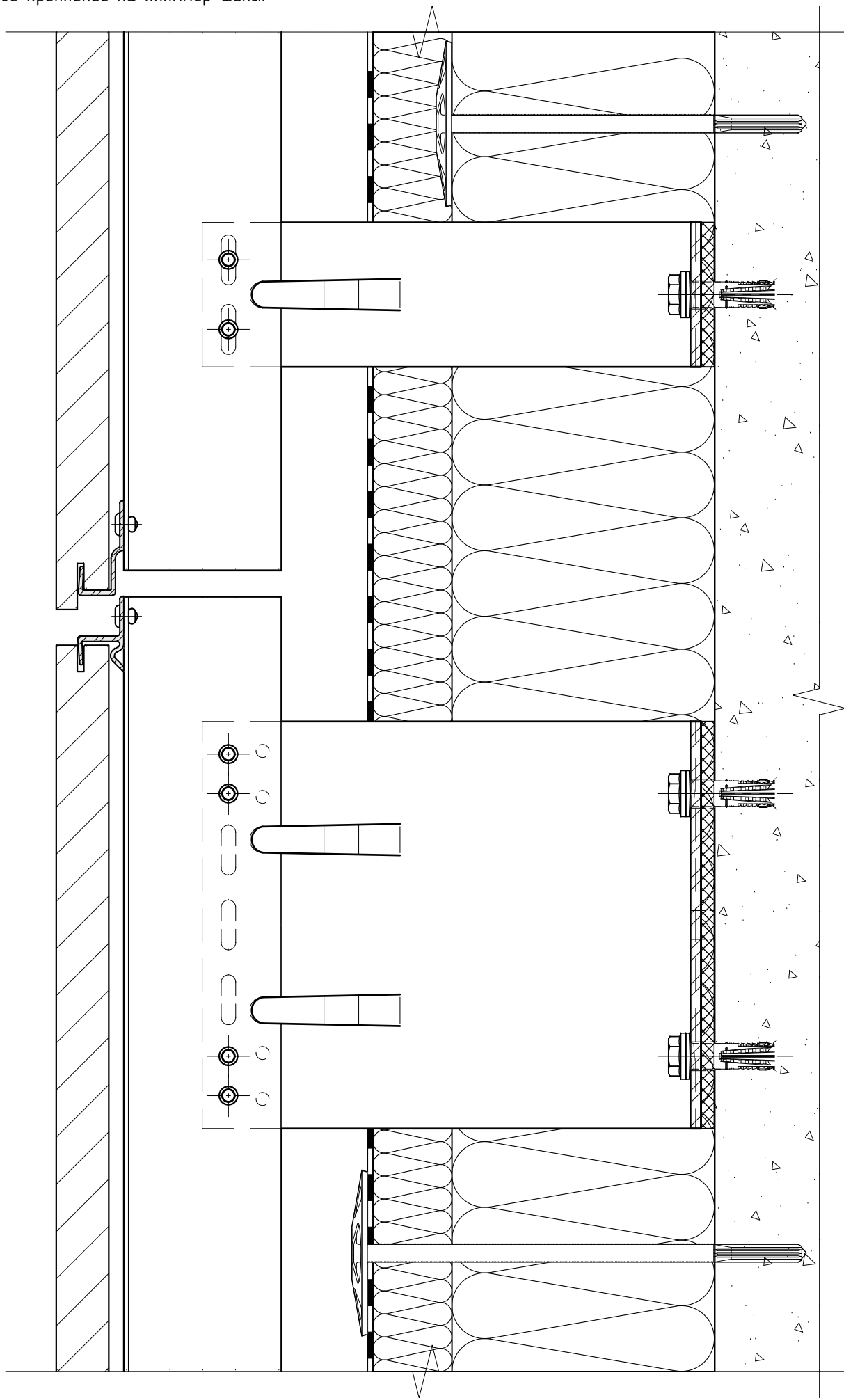
Фрагмент №1 (крепление на нерж. кляммер-шины)
