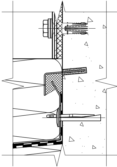
Фрагмент №1 (дополнительный вариант примыкания цоколя к НВФ в зоне строительного основания)
