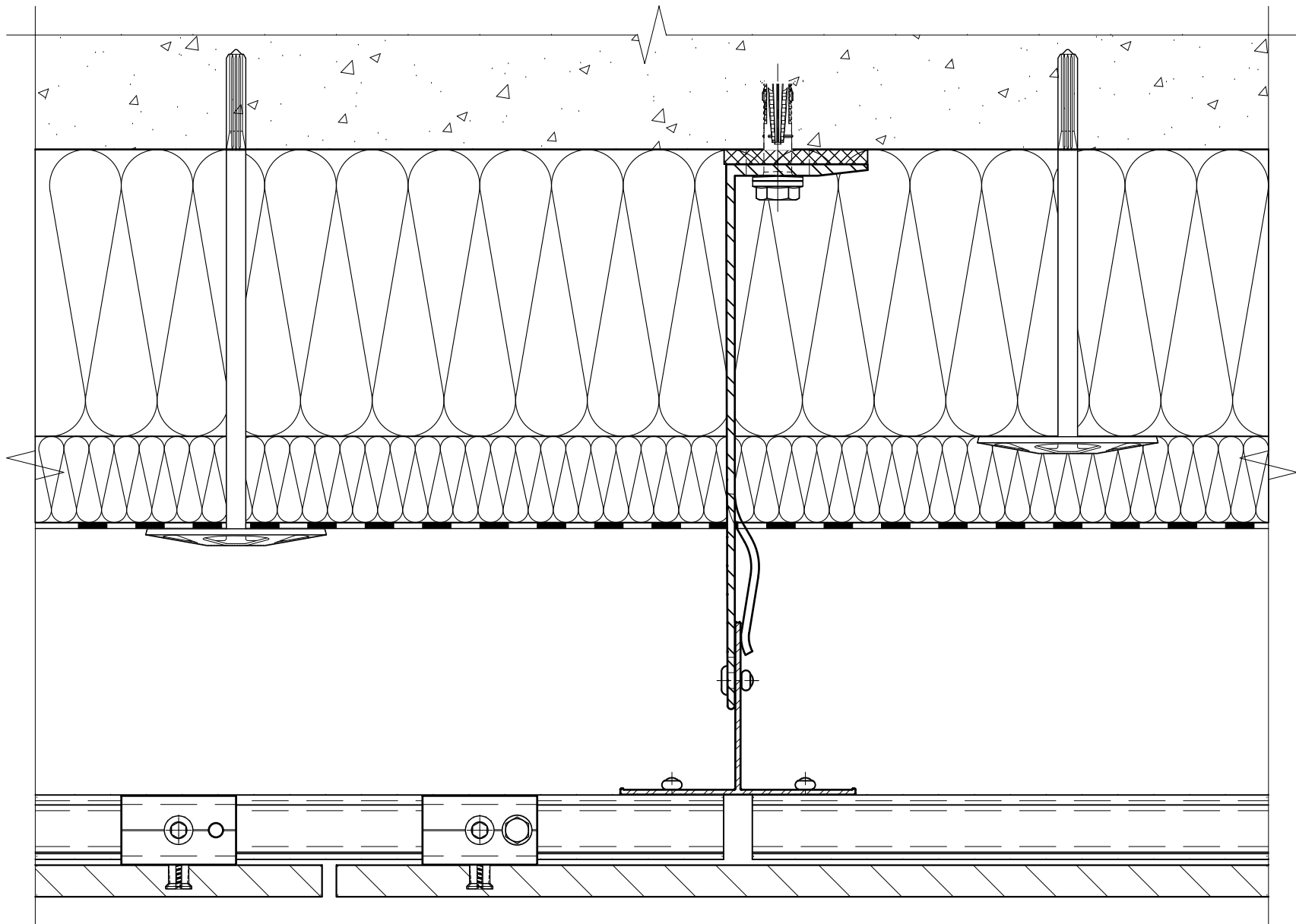
Горизонтальный разрез: элементы "Light", скрытое крепление на аграфы.
