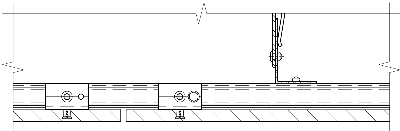
Фрагмент №1 (промежуточное крепление горизонтального профиля)
