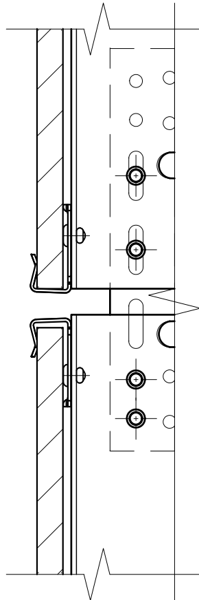
Фрагмент №1 (доп. вариант исполнения)
