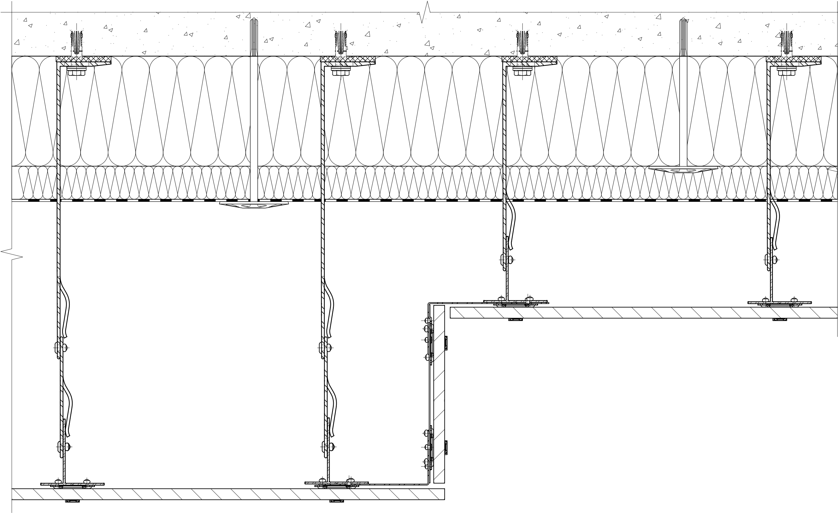
Организация перепада плоскостей облицовки: горизонтальный разрез, видимое крепление на кляммера, вариант №1.
