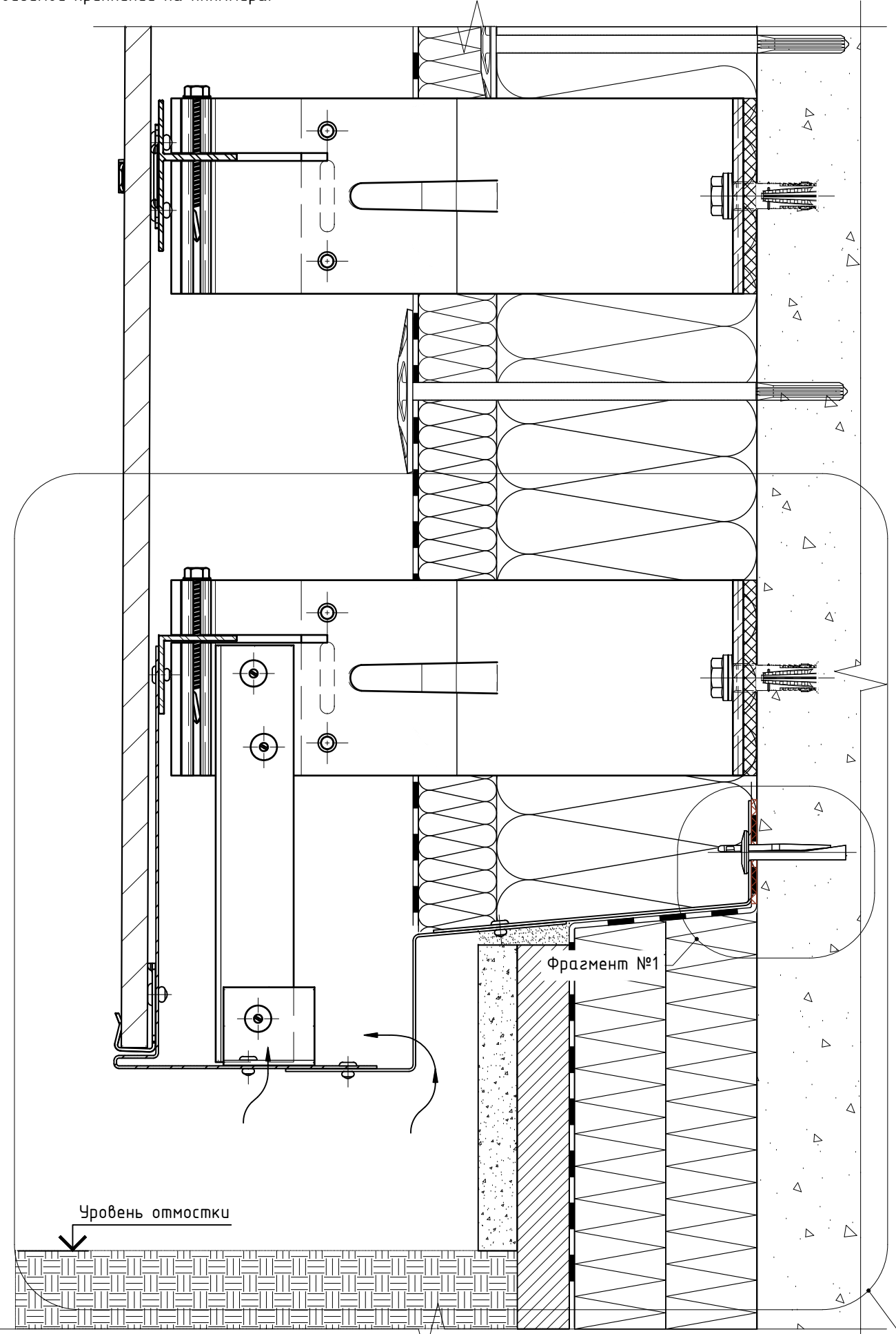
Фрагмент №1 (дополнительный вариант примыкания цоколя к НВФ в зоне строительного основания)
