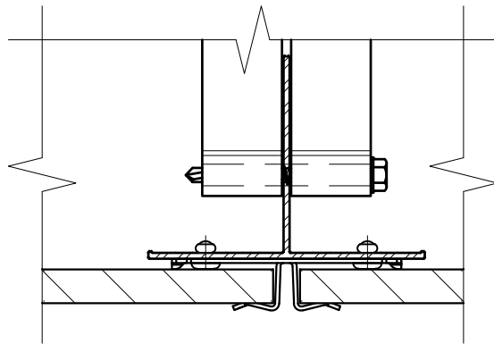
Фрагмент №1 (промежуточное крепление плиты по вертикальному шву облицовки, дополнение к стандартным решениям для площадок с расчетной сейсмичностью 7 и более баллов)
