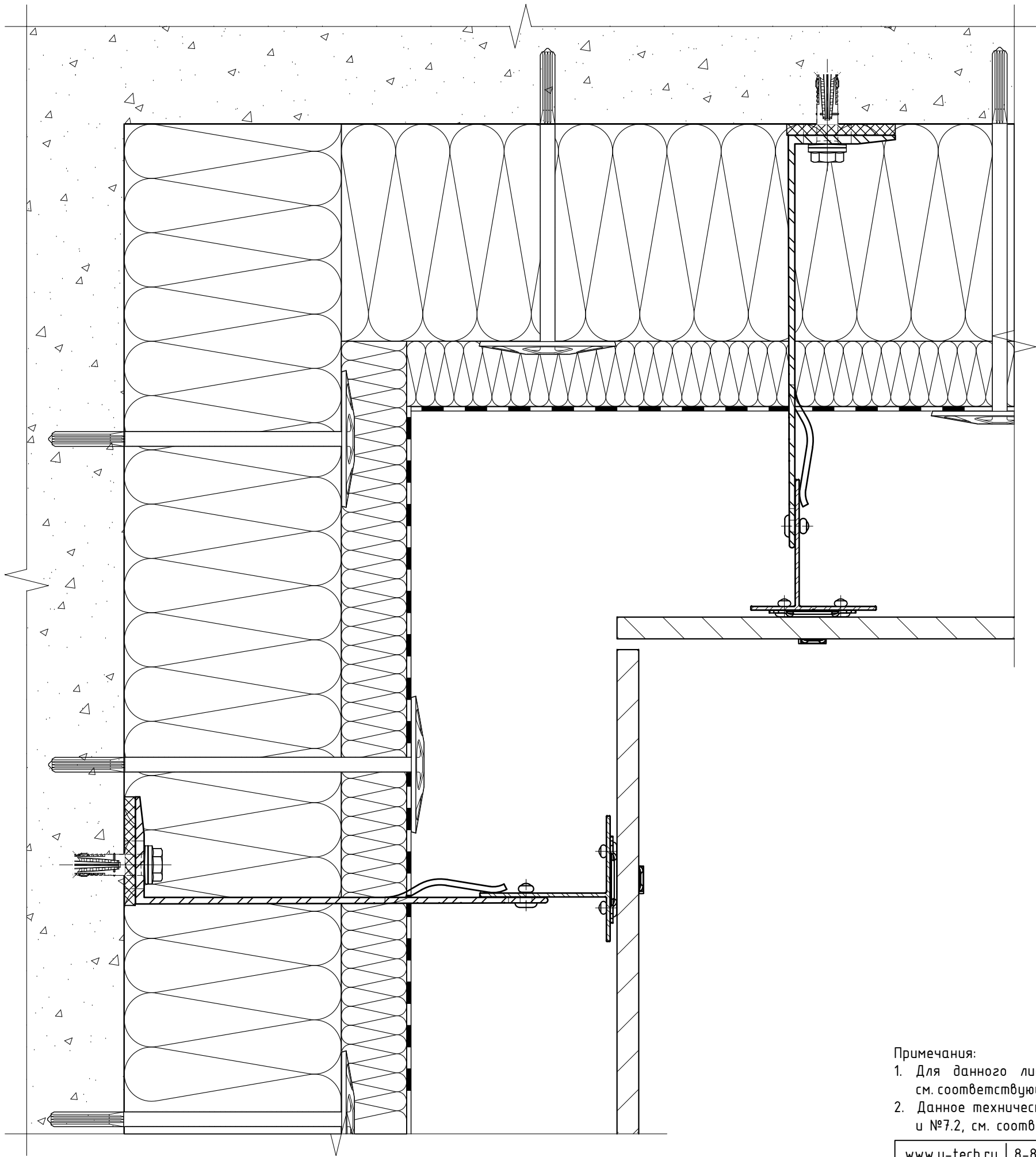
7.8. Выполнение внутреннего угла фасада: элементы "Light", вертикальная схема расположения элементов системы, видимое крепление на кляммерах.
