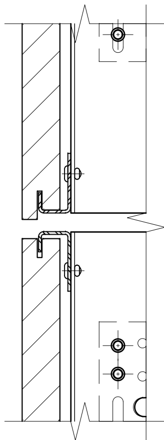
Фрагмент №1 (крепление на нерж. кляммер-шины)
