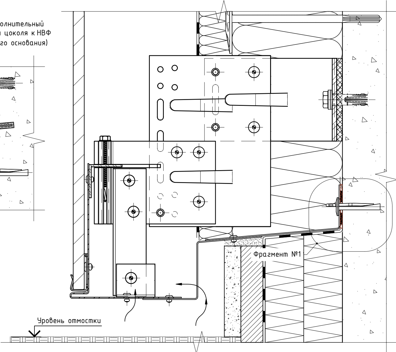
Фрагмент №2 (доп.вариант компоновки нижнего крепления к стр.основанию)
