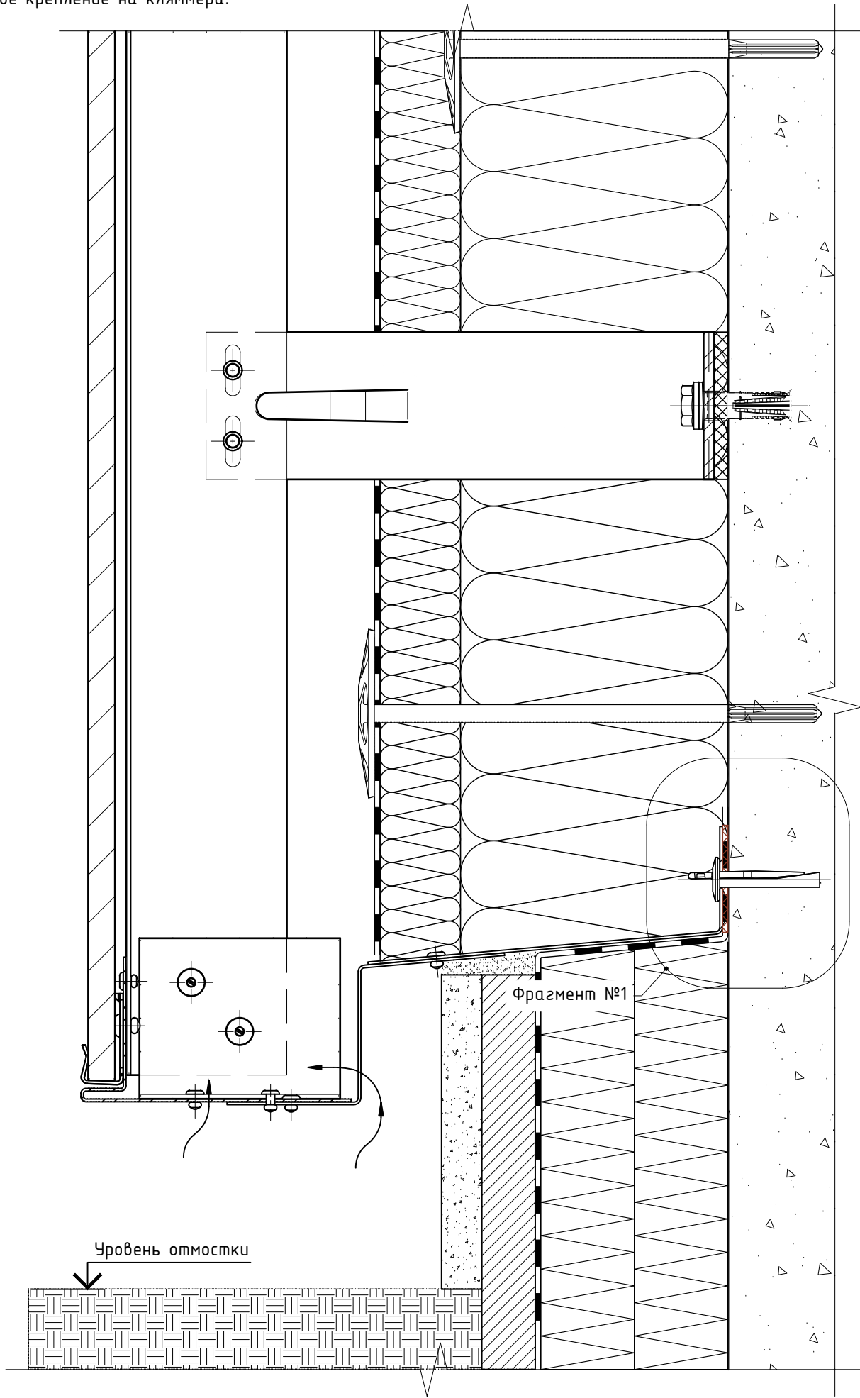
Фрагмент №1 (дополнительный вариант примыкания цоколя к НВФ в зоне строительного основания)
