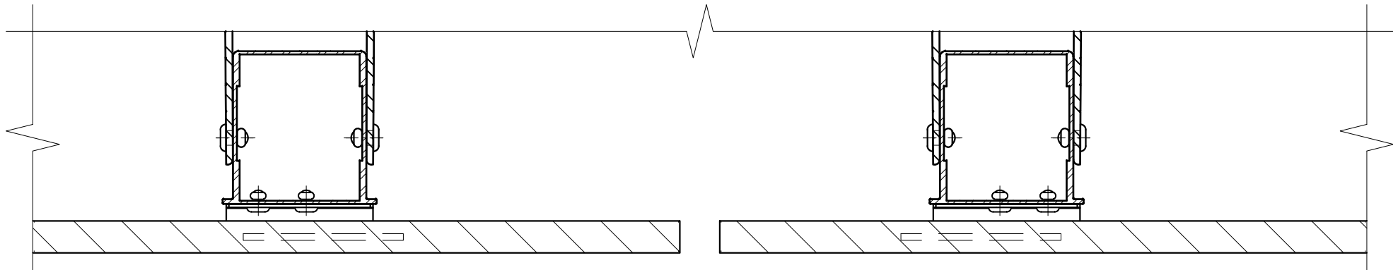
Фрагмент №1 (элементы "Heavy", скрытое крепление на кляммера (в пропилы))
