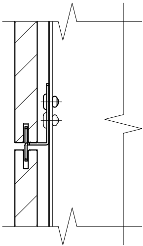
Фрагмент №1 (промежуточное крепление плиты по горизонтальному шву облицовки вне зоны стыковки вертикальных направляющих)
