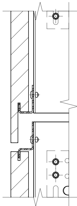
Фрагмент №1 (доп. вариант крепления на нерж. кляммер-шины)
