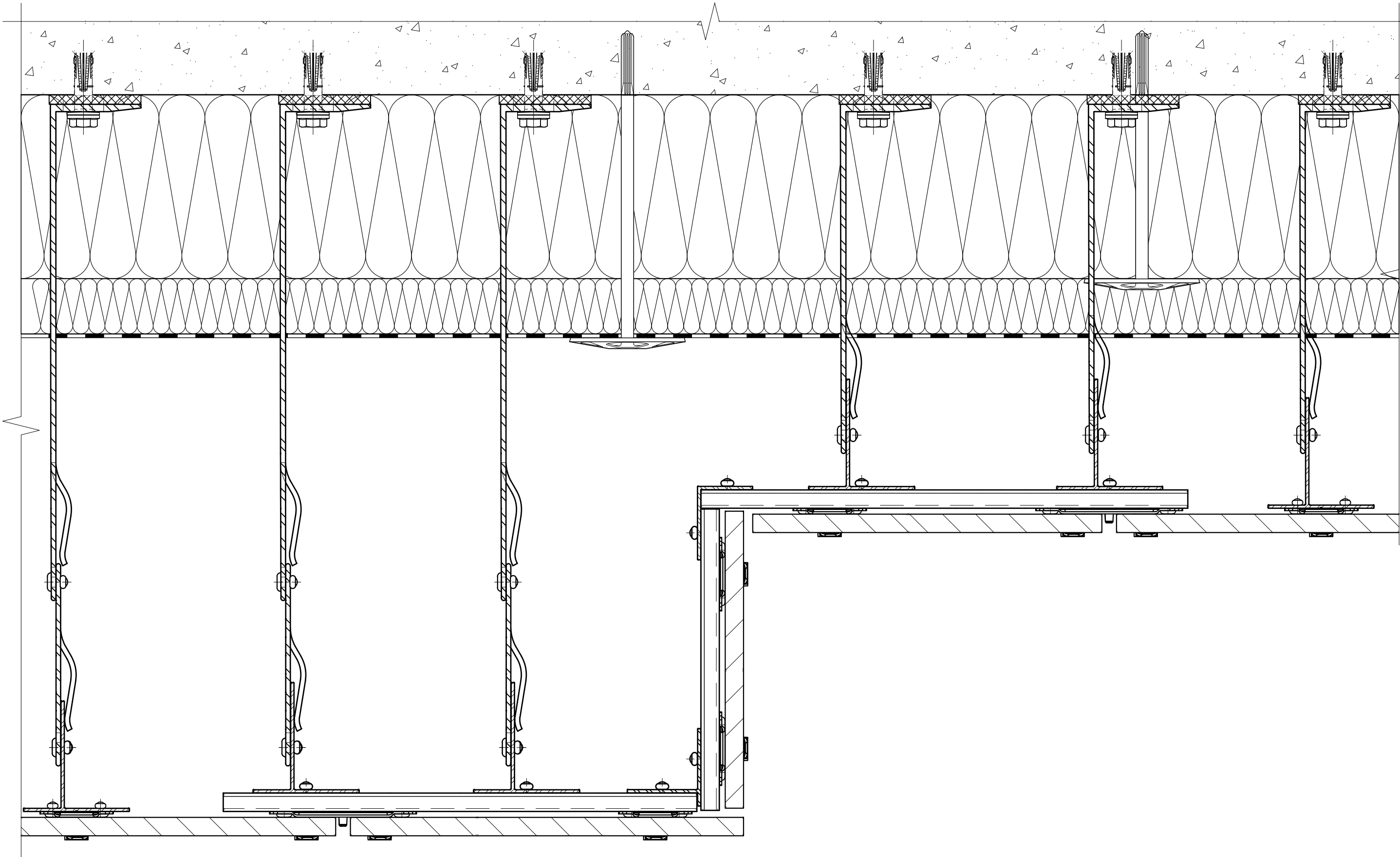
Организация перепада плоскостей облицовки: горизонтальный разрез, видимое крепление на кляммера, вариант №2.
