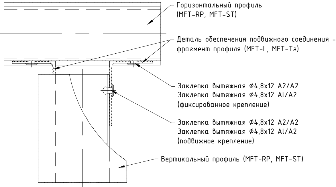
Узел №2 (увеличено)
