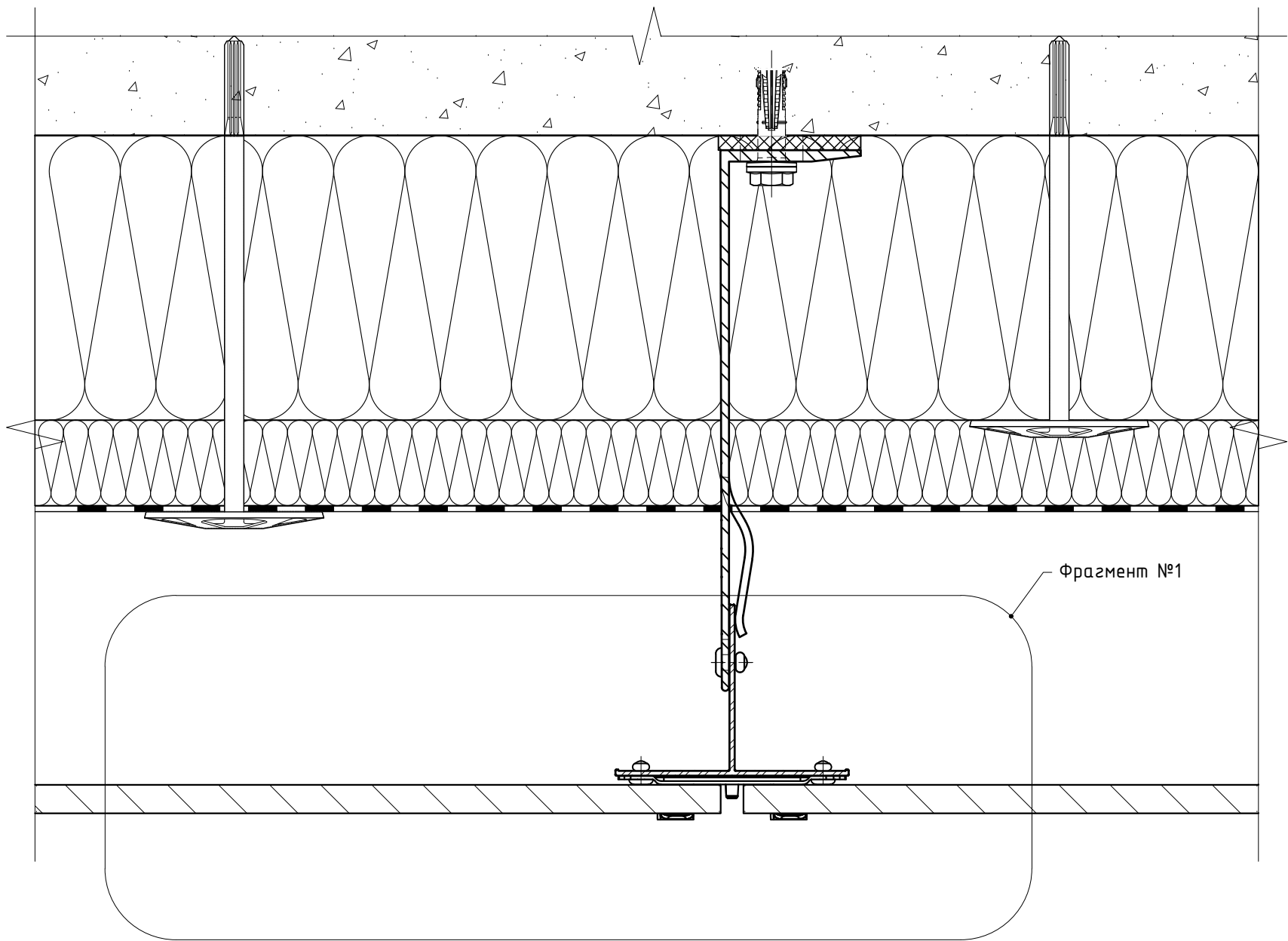
Фрагмент №1 (промежуточное крепление плиты по вертикальному шву облицовки, дополнение к стандартным решениям для площадок с расчетной сейсмичностью 7 и более баллов)
