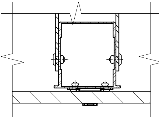
Фрагмент №1 (промежуточное крепление плиты по горизонтальному шву облицовки)
