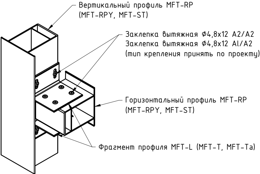
Узел №5 (увеличено)
