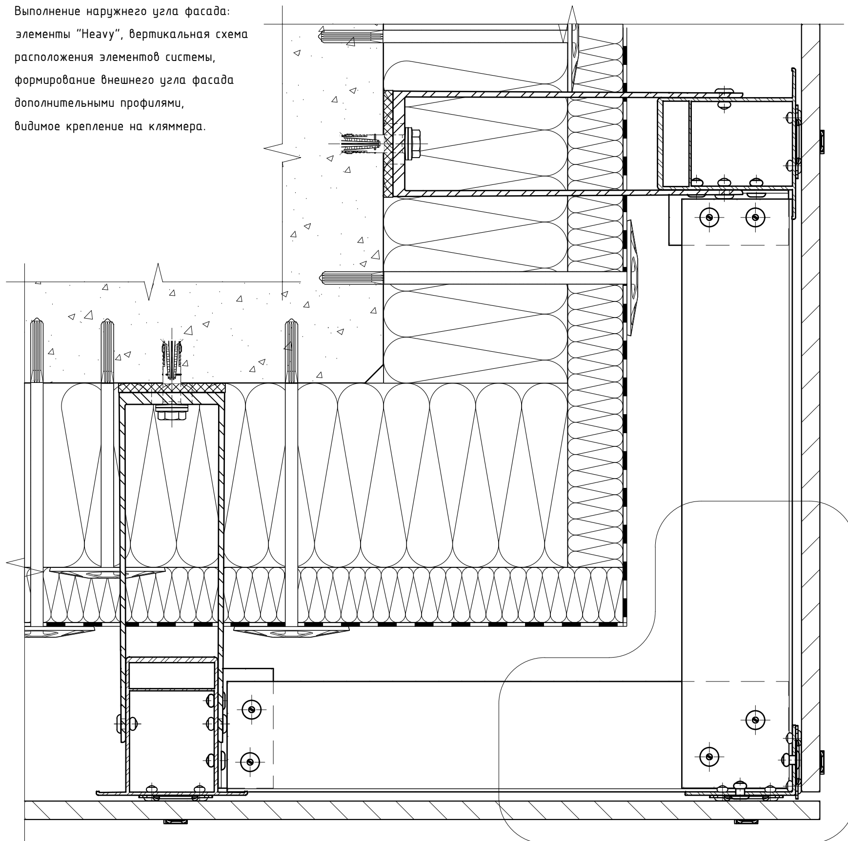
Фрагмент №1
