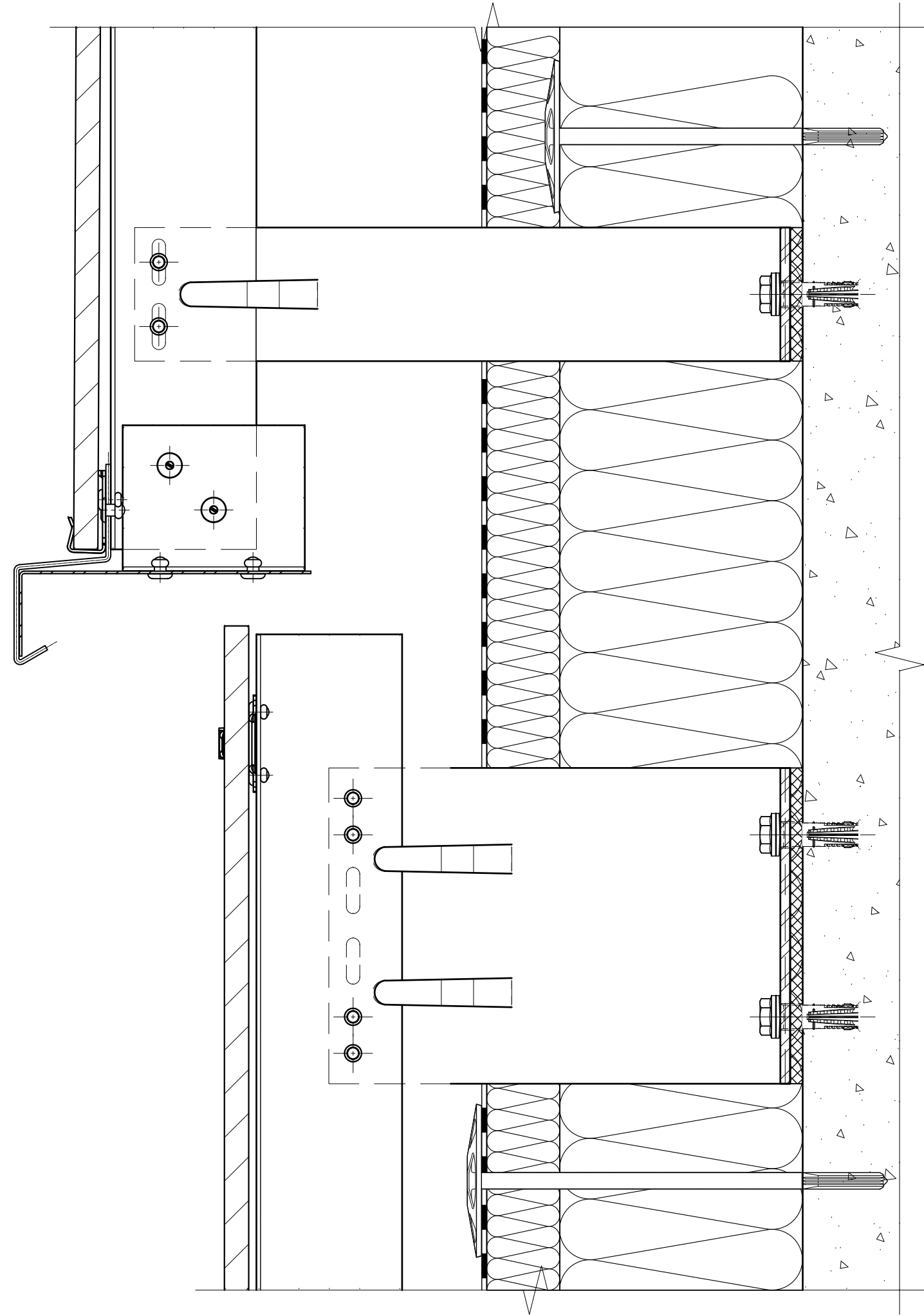
Организация перепада плоскостей облицовки: вертикальный разрез, видимое крепление на кляммера, вариант №2.
