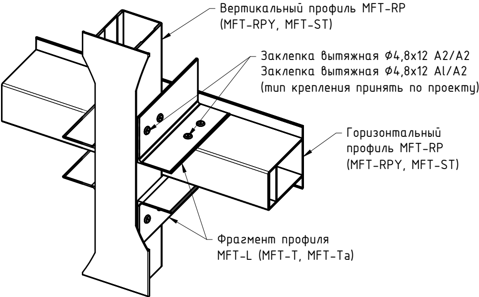
Узел №4 (увеличено)
