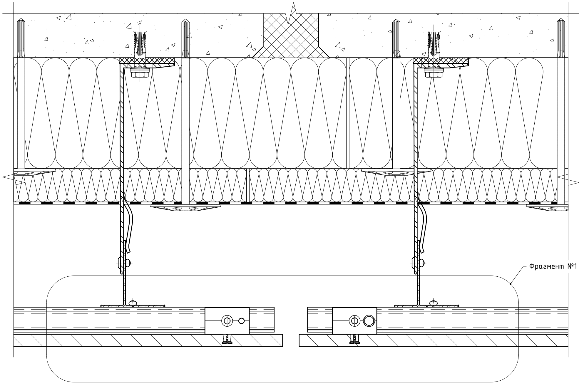
Фрагмент №1 (элементы "Heavy", скрытое крепление на кляммер-шины)
