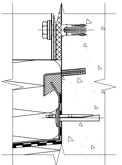
Фрагмент №1 (дополнительный вариант примыкания цоколя к НВФ в зоне строительного основания)
