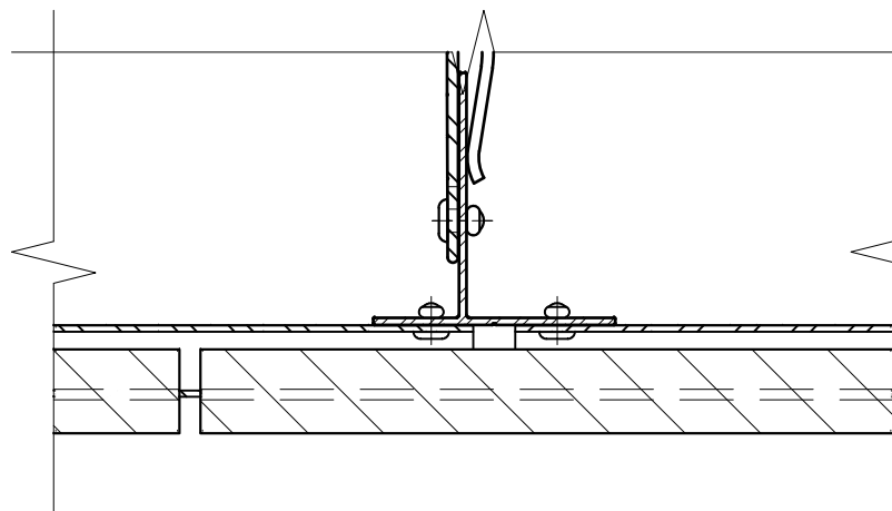
Фрагмент №1 (крепление на нерж. кляммер-шины)
